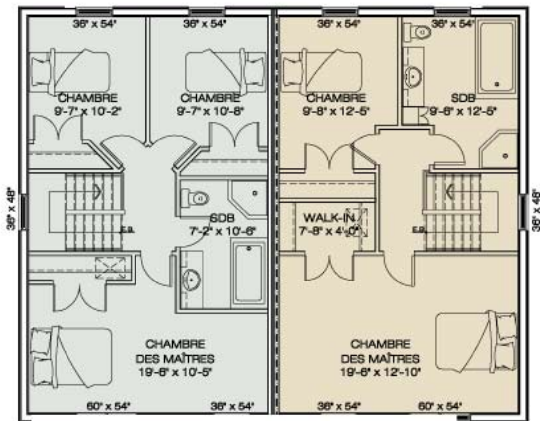
PLAN DE L'ÉTAGE CONDO 2 CHAMBRES
